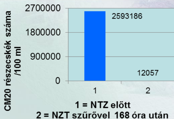
Részecskék > 2 mikron
