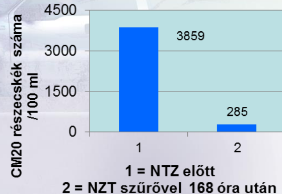
Részecskék > 15 mikron
