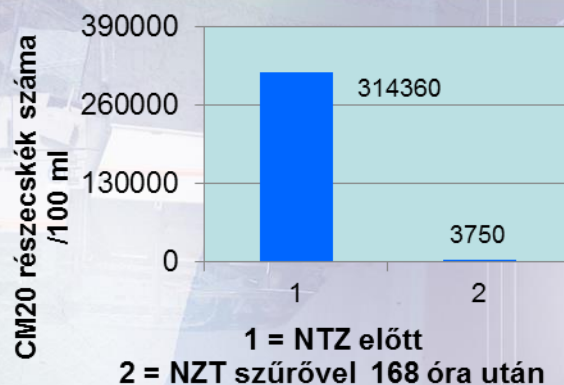
Részecskék > 5 mikron
